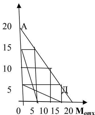
Рис. 9.2. График соотношения M_{УПП} и M_{отх}
